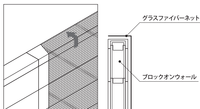
片面工場塗装の場合
