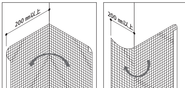
入隅部(回し張り)
