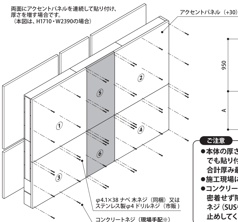
レイアウト例 (H1710・W2390の場合)
